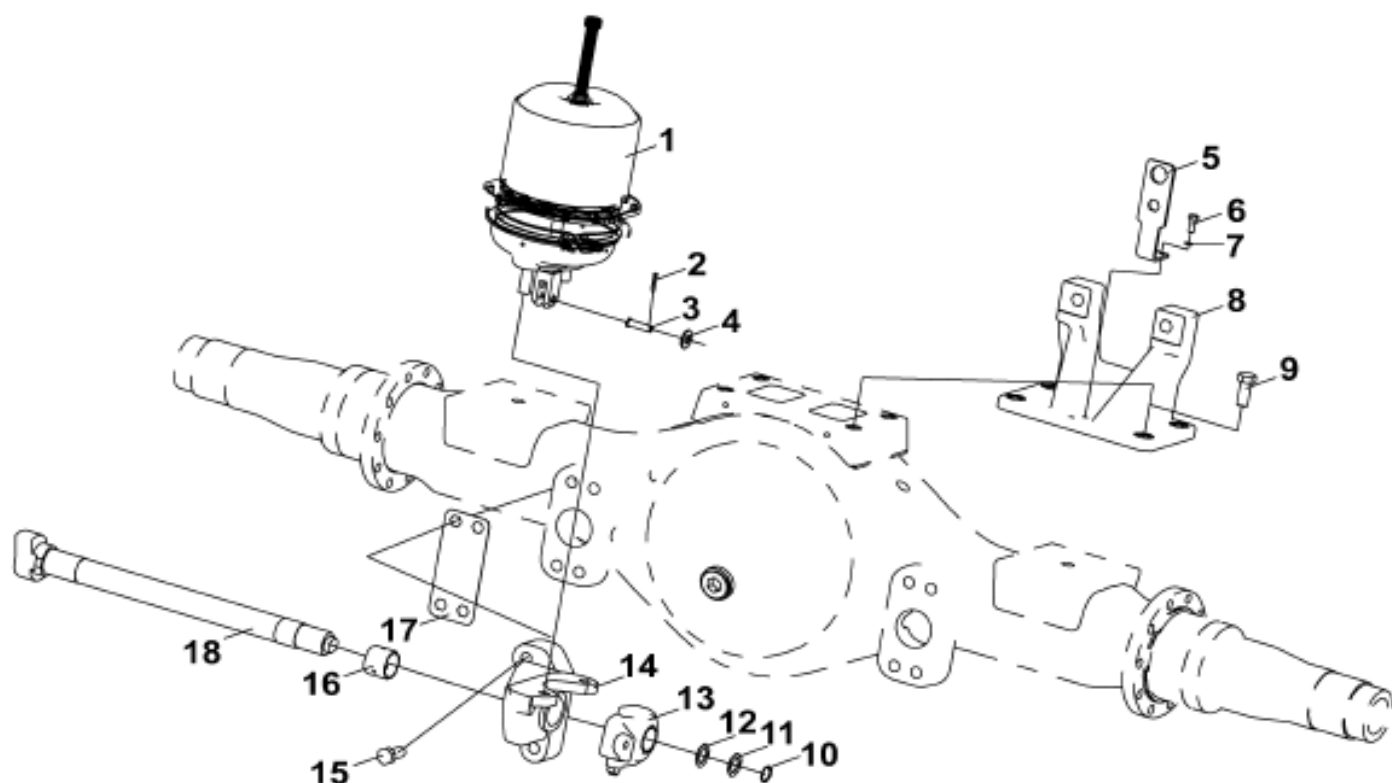
Рис.157. Привод тормозов заднего моста
