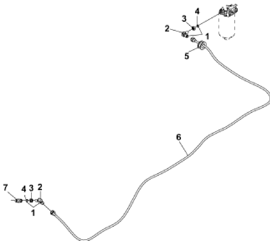
Рис.63. Магистраль подачи топлива
