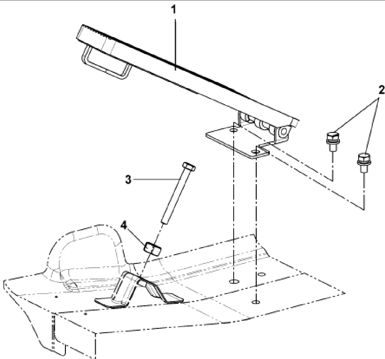
Рис.218. Педаль акселератора
