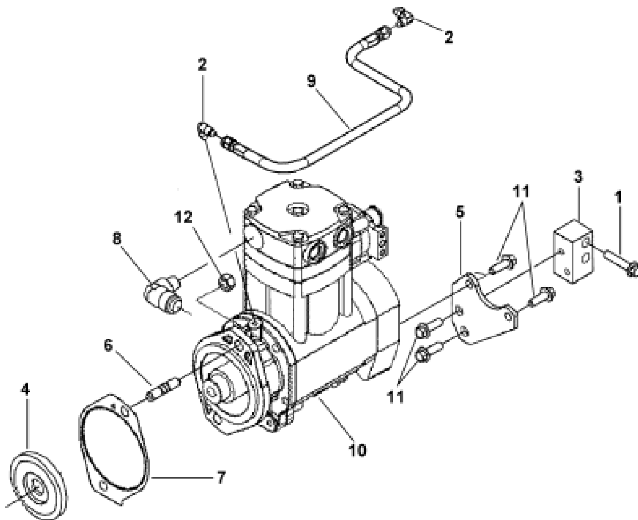
Рис.33. Компоновка компрессора
