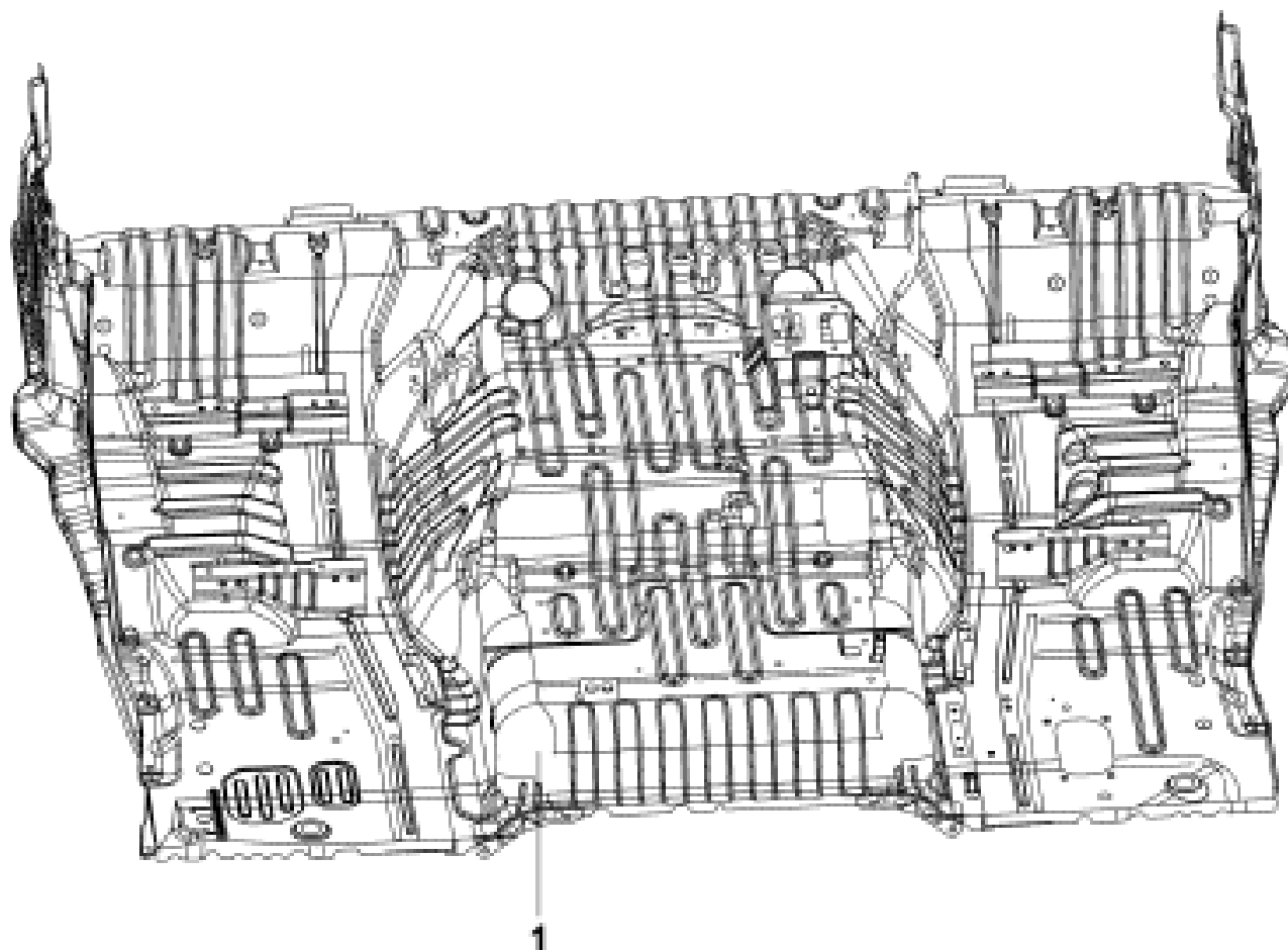
Рис.285. Панель пола в сборе
