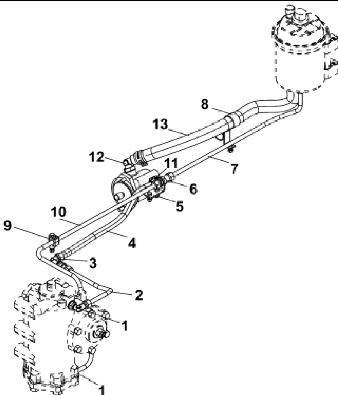
Рис.185. Трубопровод гидроусилителя
