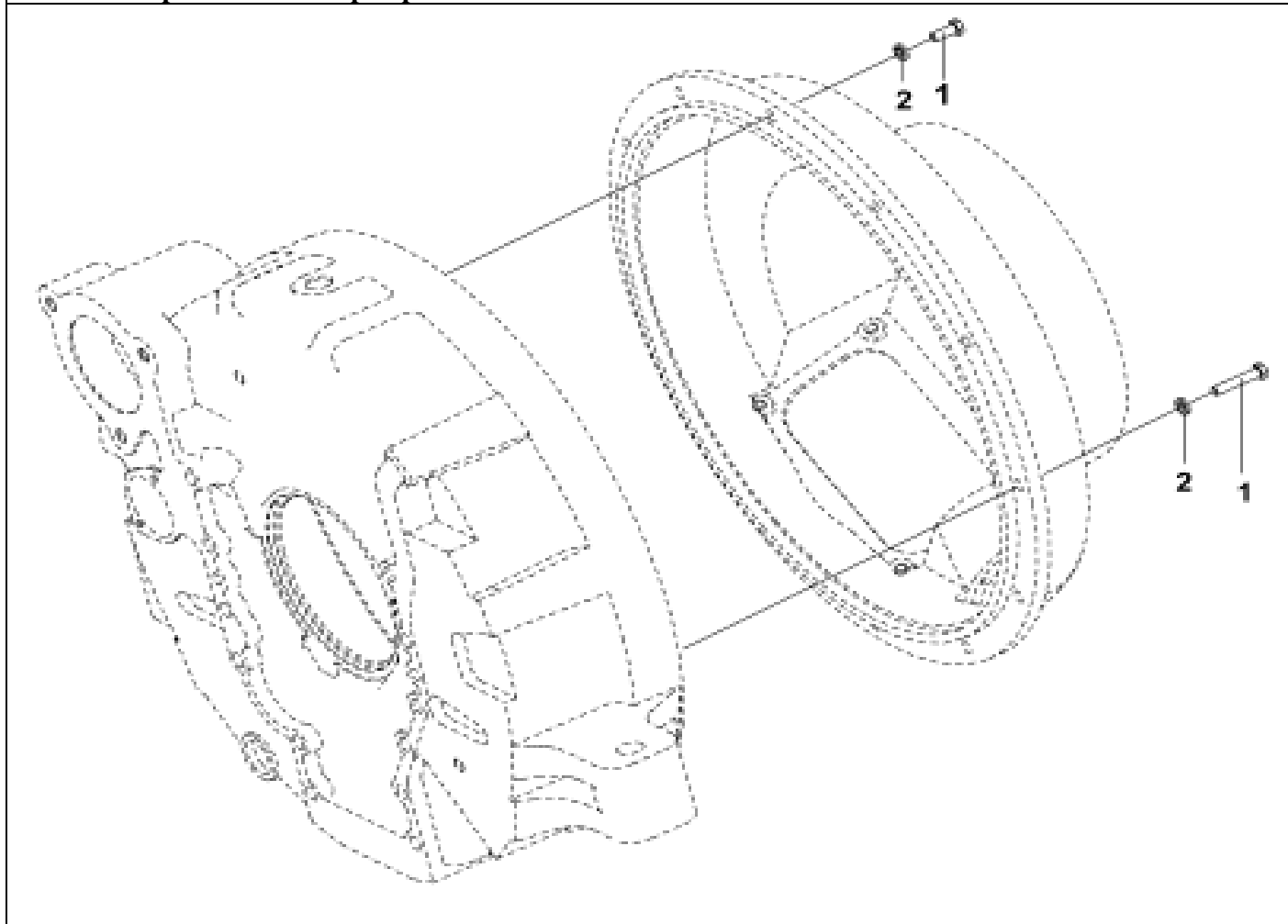
Рис.91. Крепление картера сцепления
