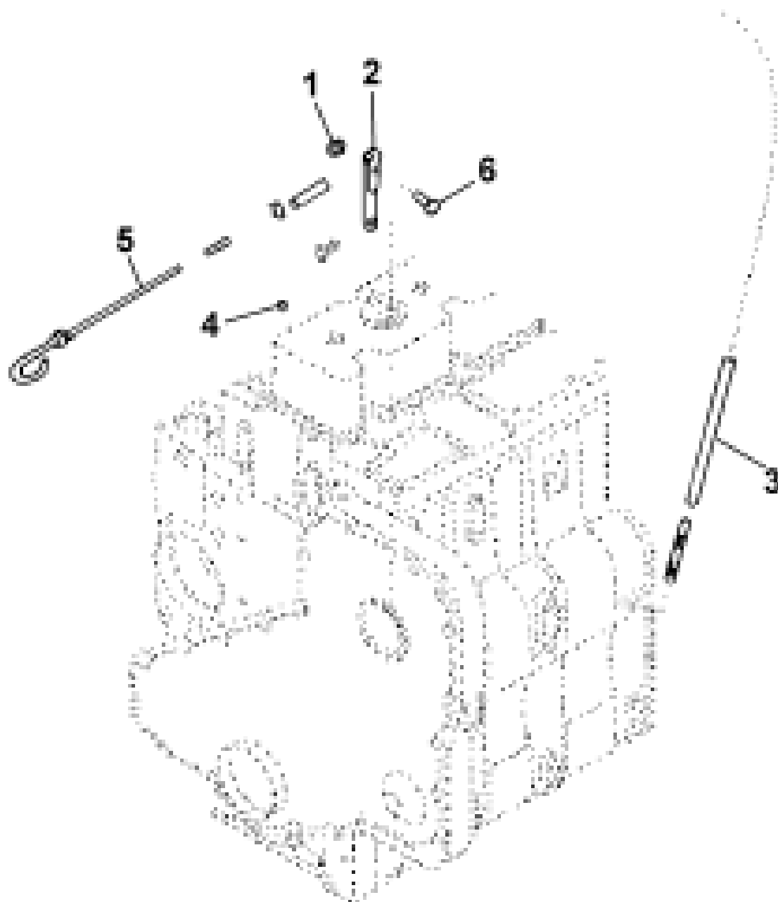
Рис.22. Масляный щуп
