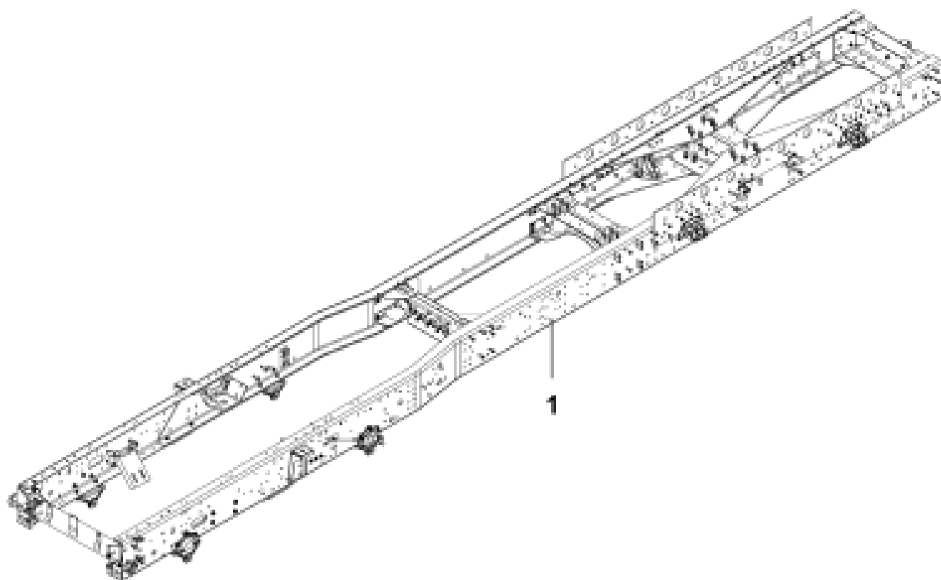
Рис.125. Рама
