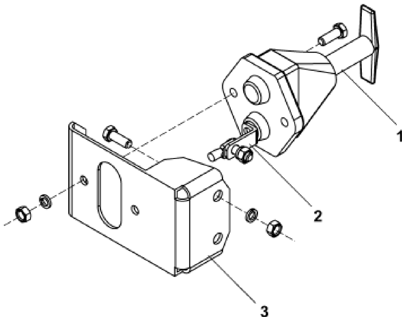
Рис.206. Выключатель массы
