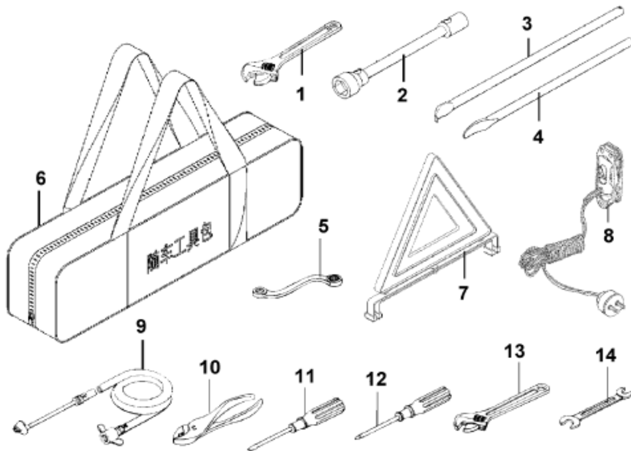
Рис.216. Сумка инструментальная
