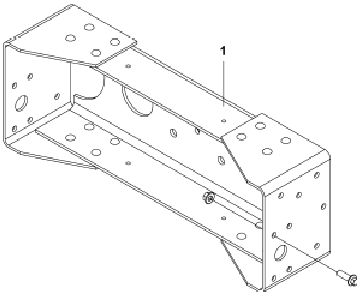
Рис.130. Буксирная поперечина
