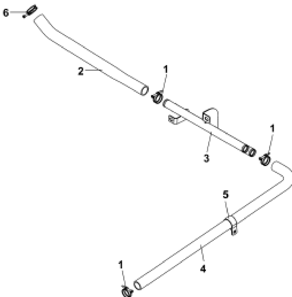
Рис.71. Трубопровод компрессора
