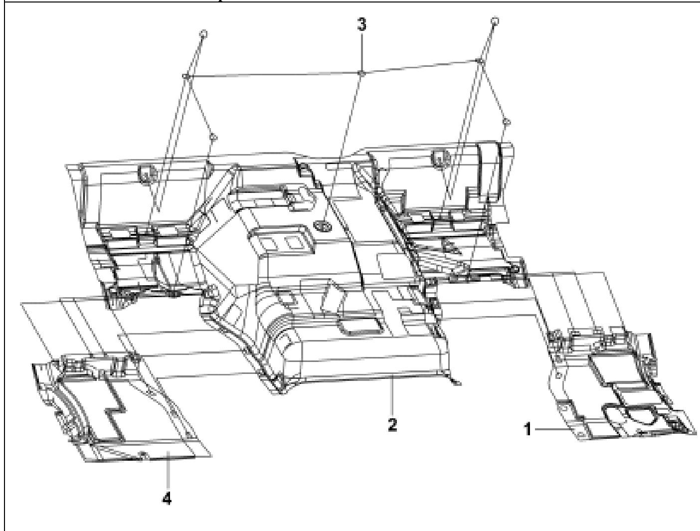
Рис.292. Напольный коврик кабины
