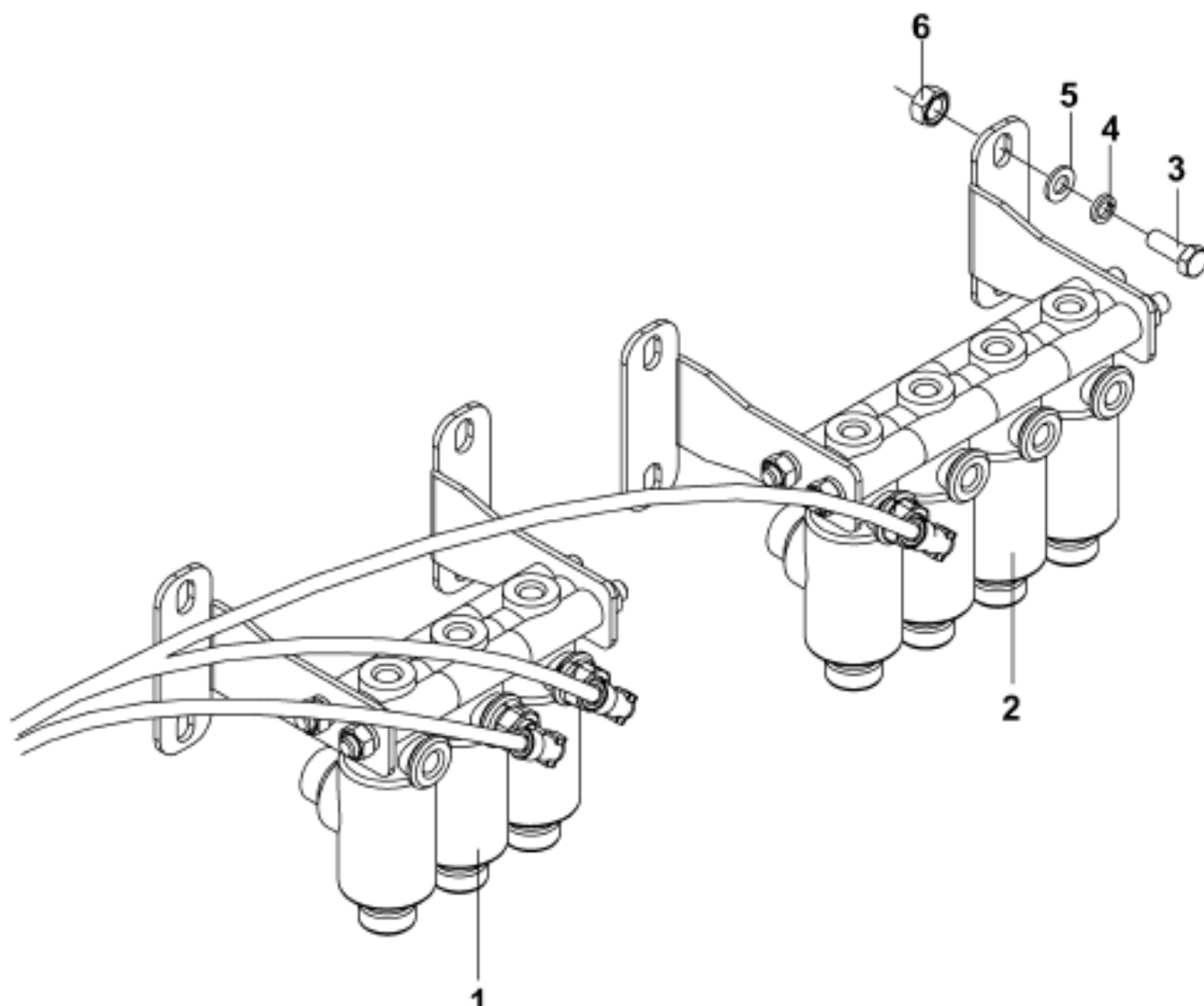
Рис.207. Блок электропневмоклапанов
