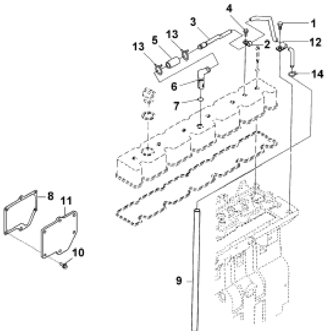
Рис.6. Вентиляция картера
