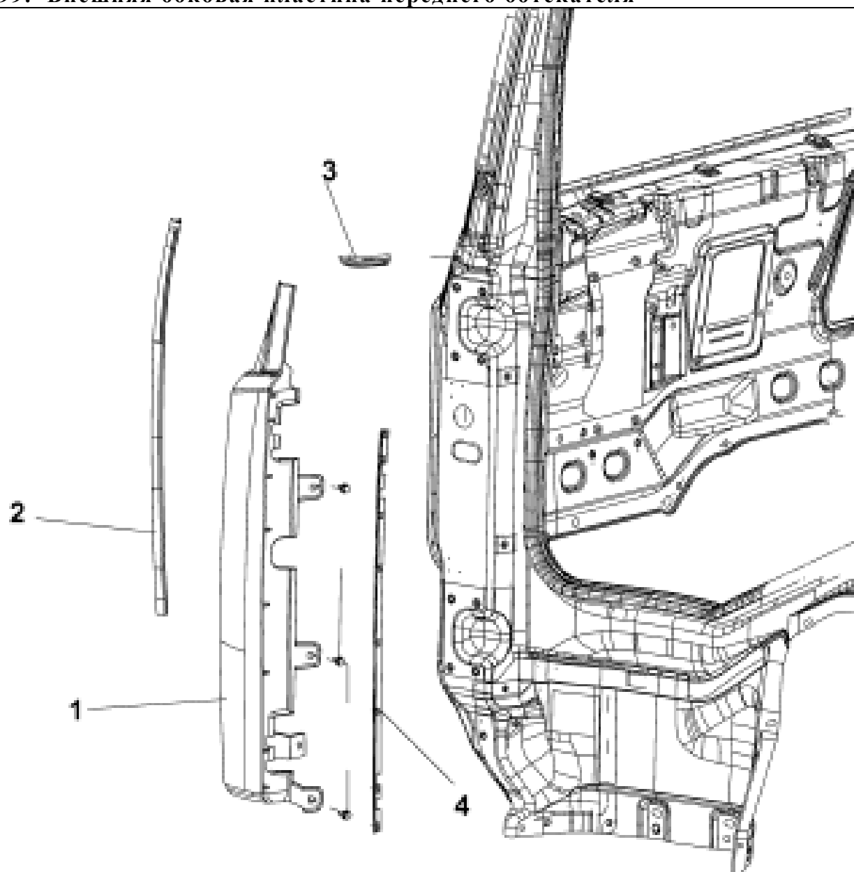
Рис.299. Внешняя боковая пластина переднего обтекателя
