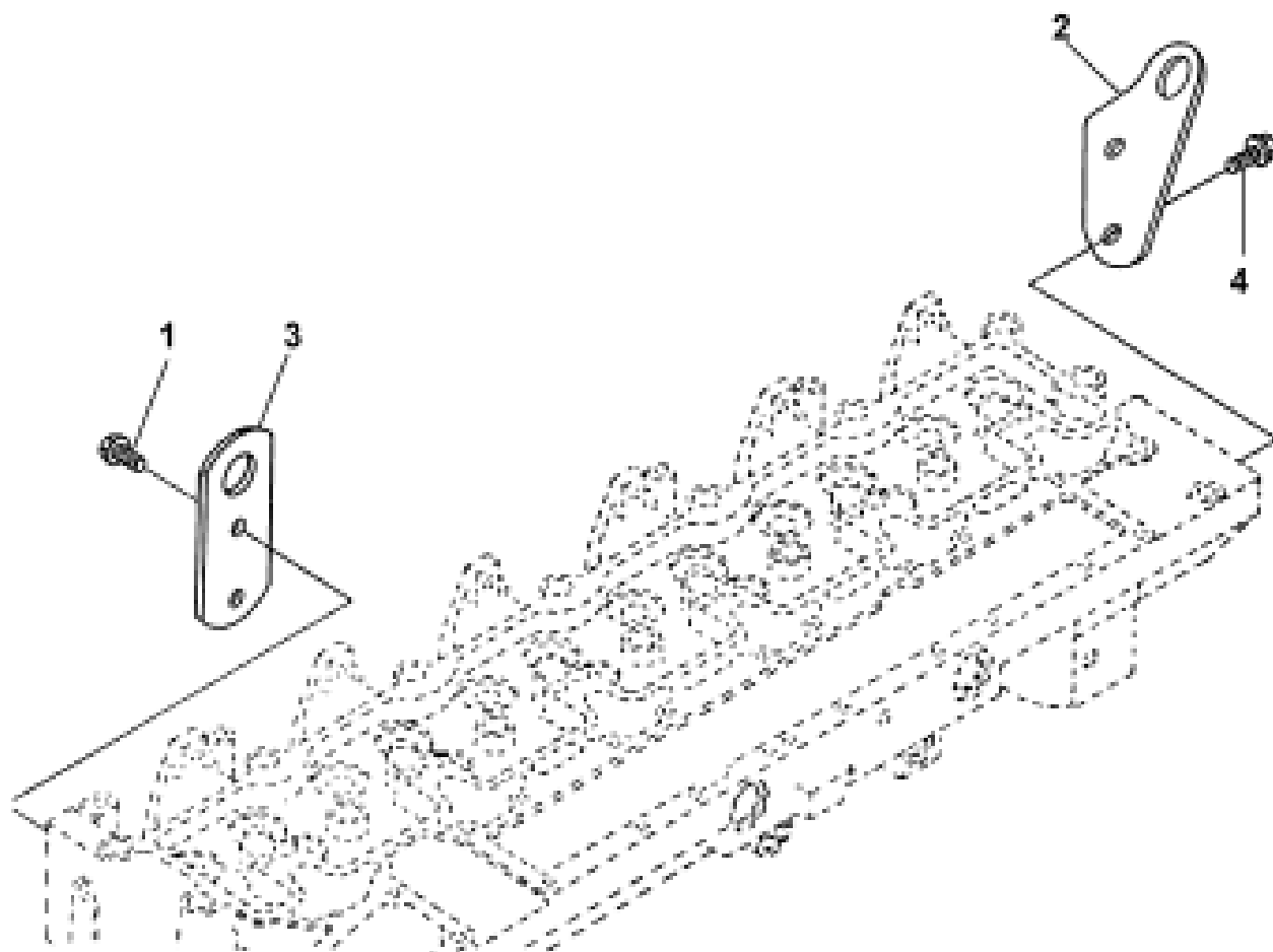
Рис.53. Серьга подвески двигателя
