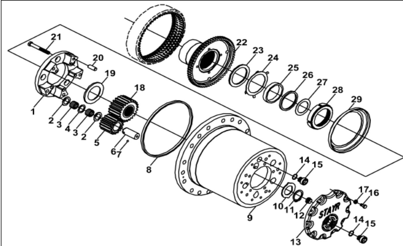
Рис.155. Колёсный редуктор заднего моста
