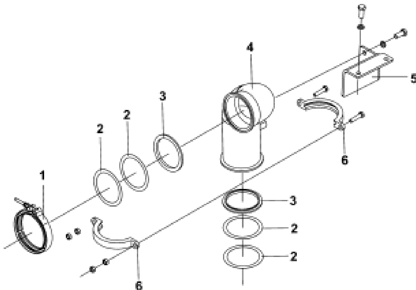
Рис.80. Соединительный патрубок турбокомпрессора
