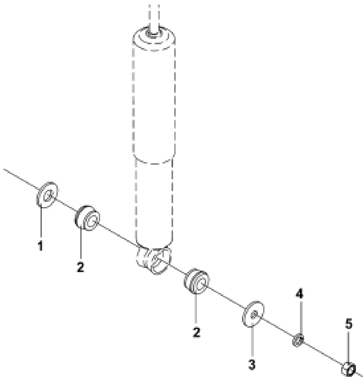
Рис.141. Нижнее крепление амортизатора
