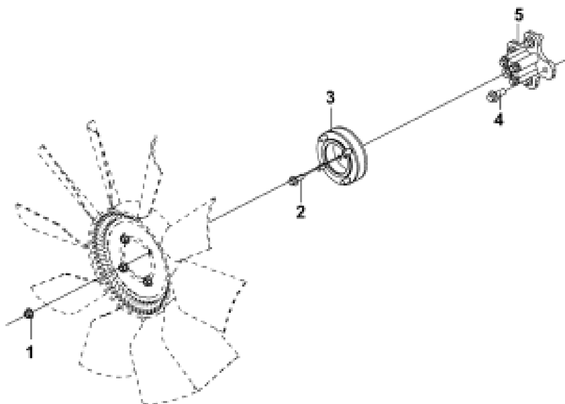
Рис.85. Установка вентилятора
