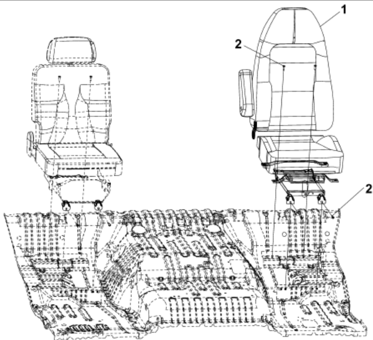
Рис.331. Сиденье водителя
