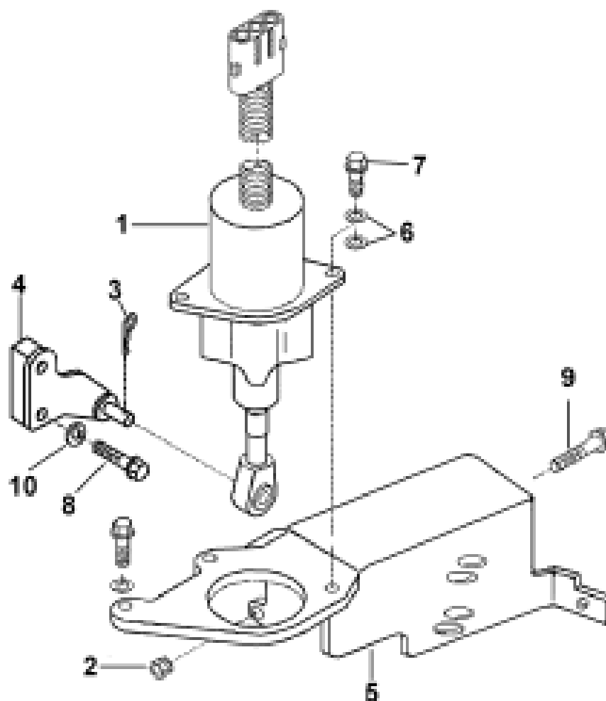
Рис.14. Установка электромагнитного клапана - отсекаателя
