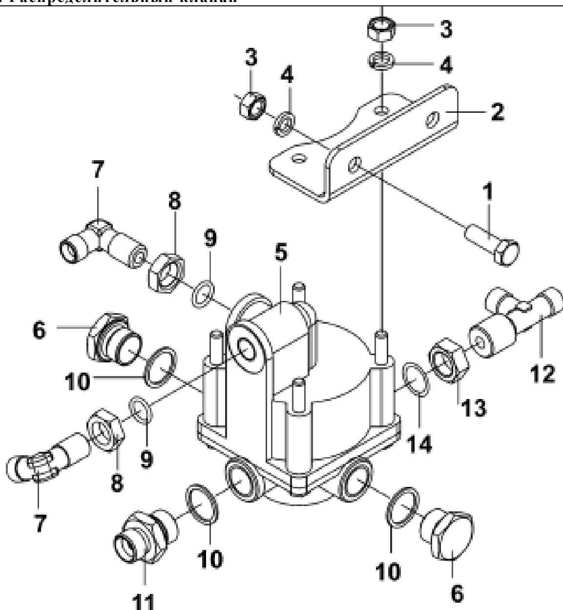
Рис.192. Распределительный клапан
