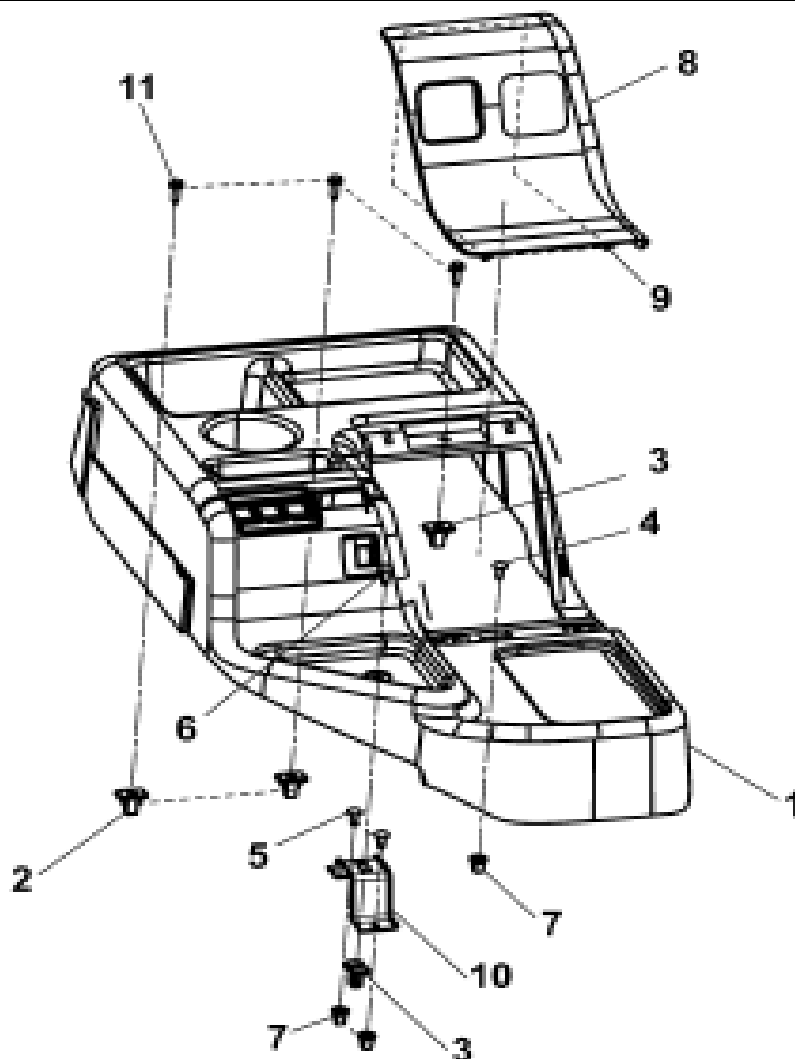
Рис.288. Вещевой ящик водителя
