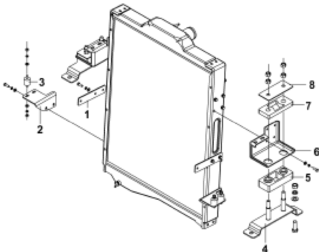
Рис.83. Крепление радиатора
