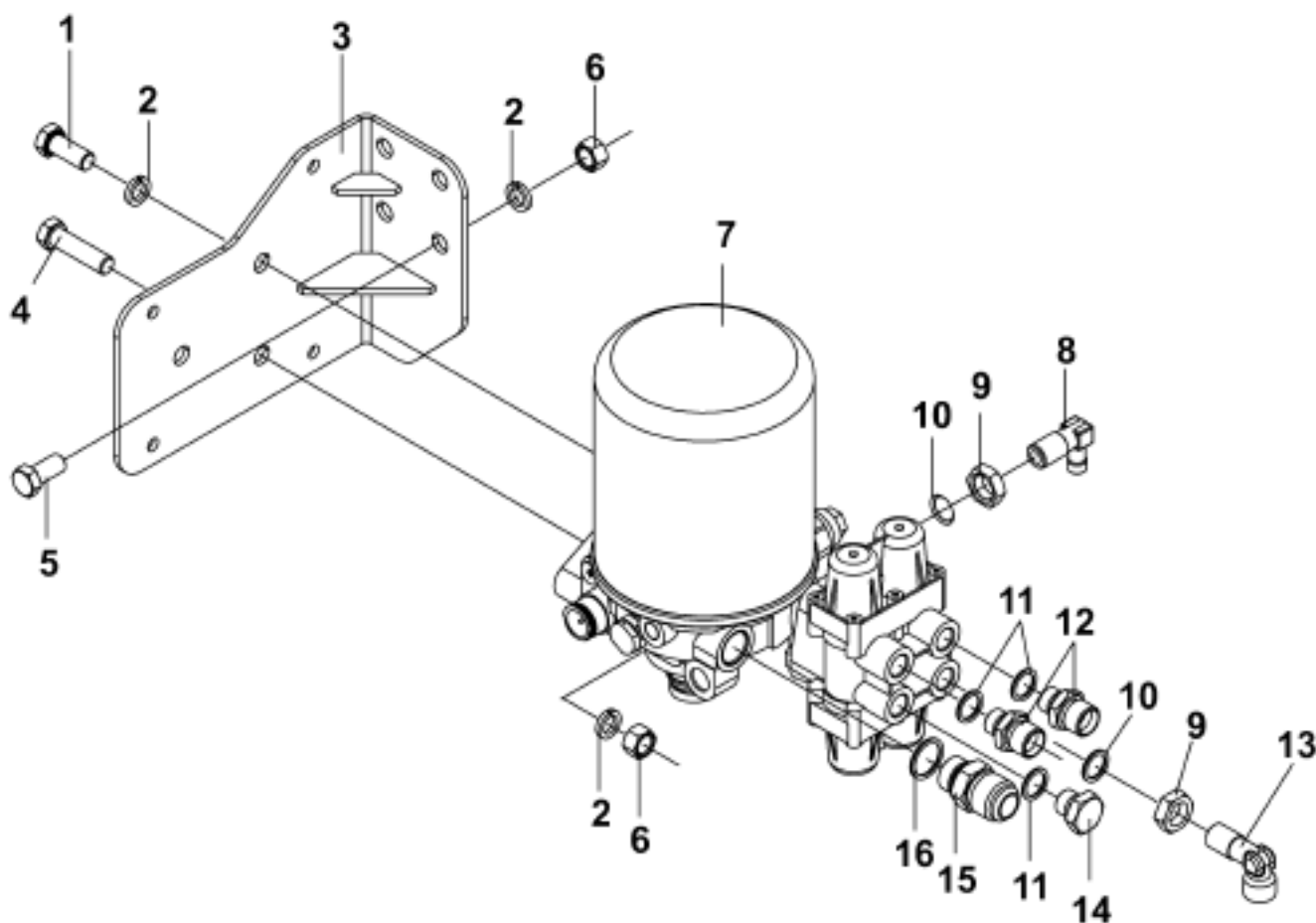
Рис.197. Влагомаслоотделитель
