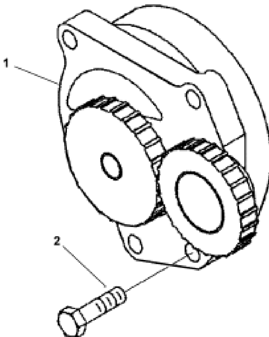
Рис.20. Масляный насос
