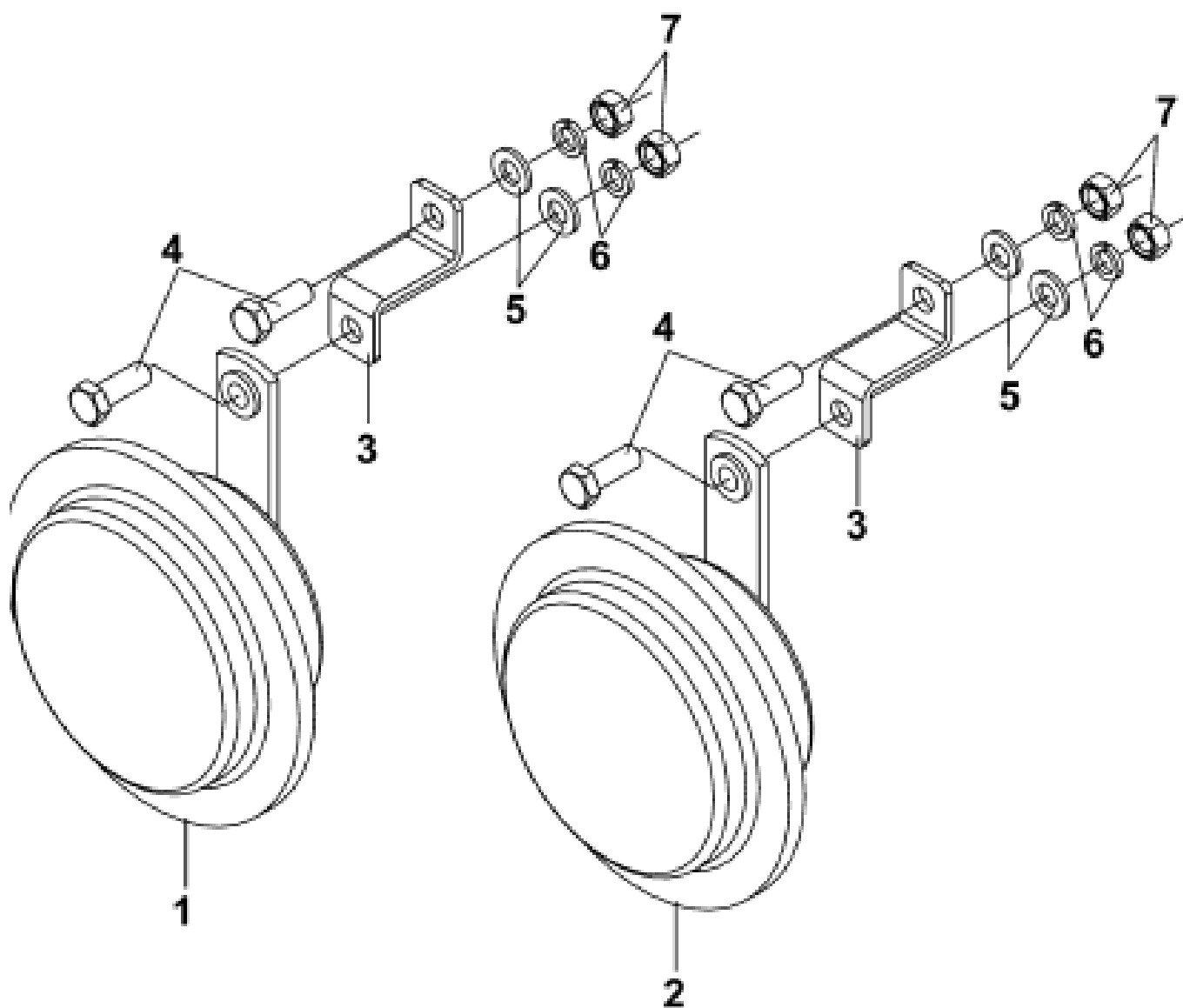
Рис.200. Электрический сигнал
