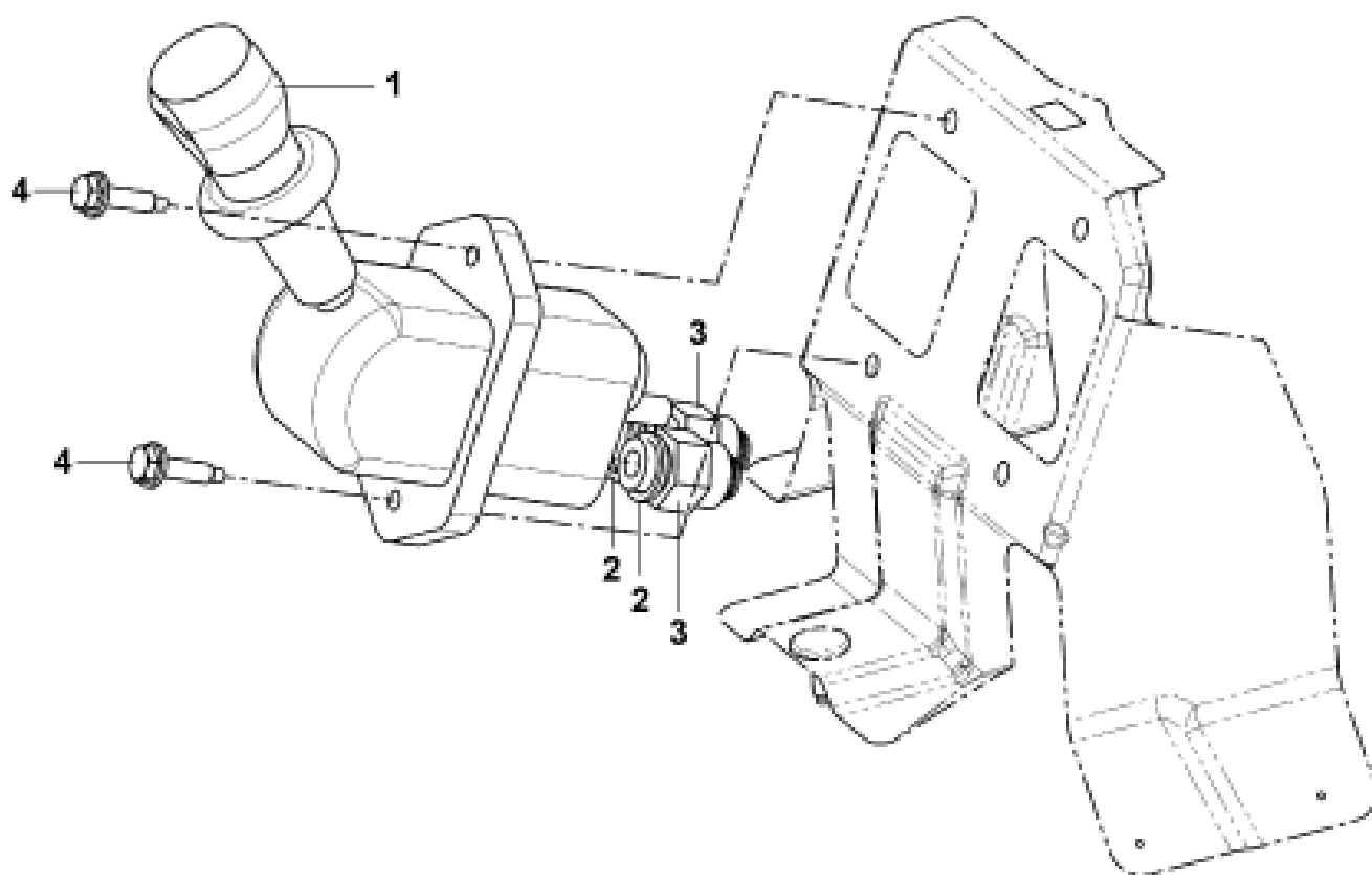
Рис.232. Установка крана ручного тормоза
