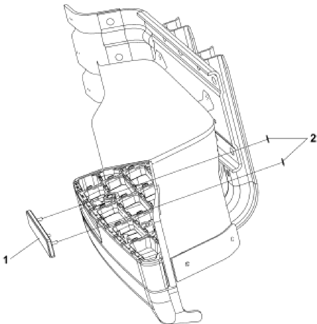
Рис.268. Отражатель
