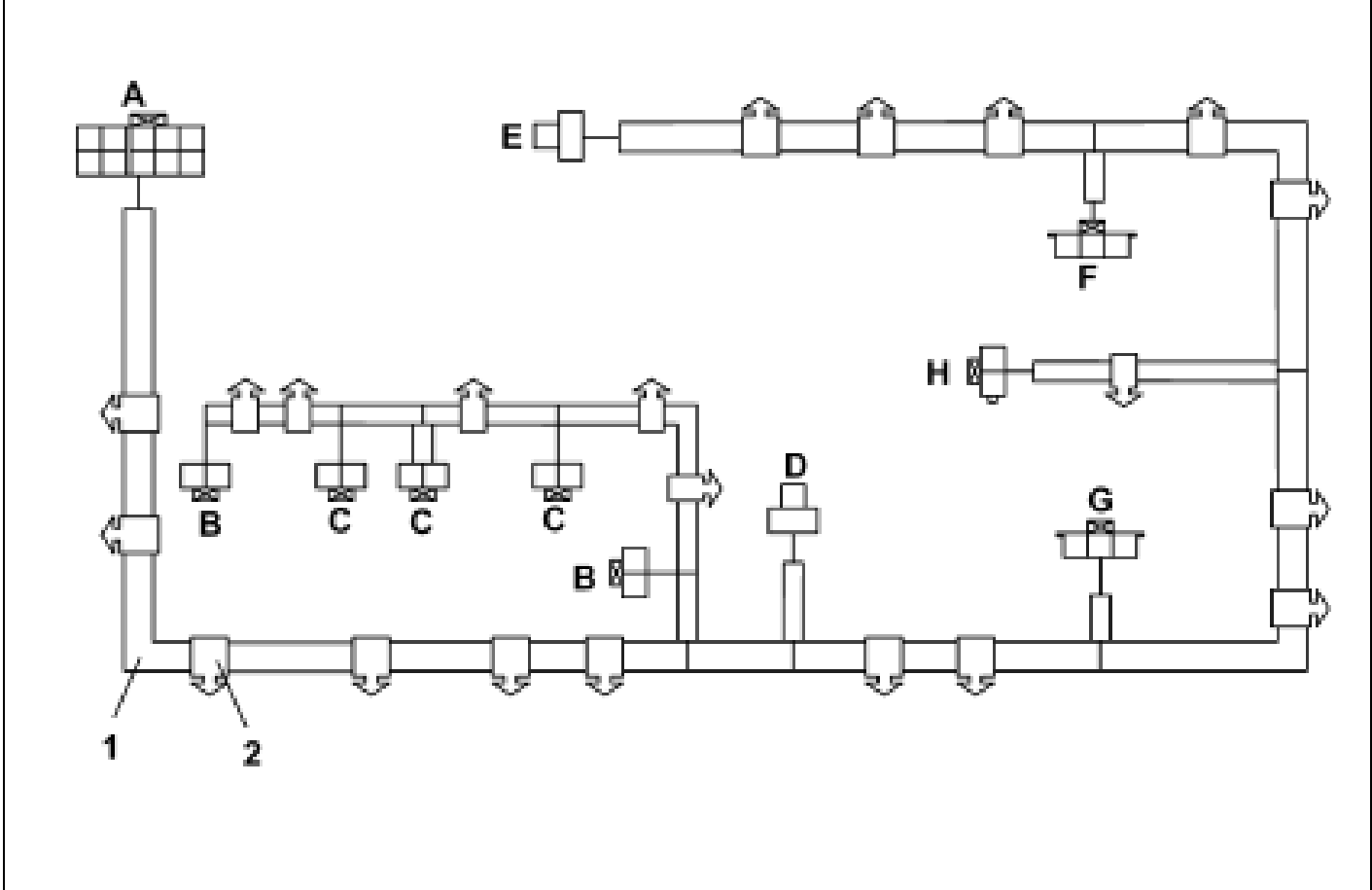
Рис.242.Схема пучка проводов потолка кабины
