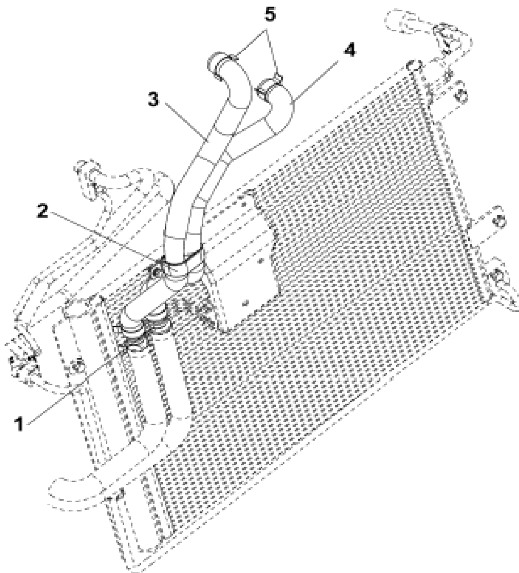
Рис.336. Радиатор отопителя
