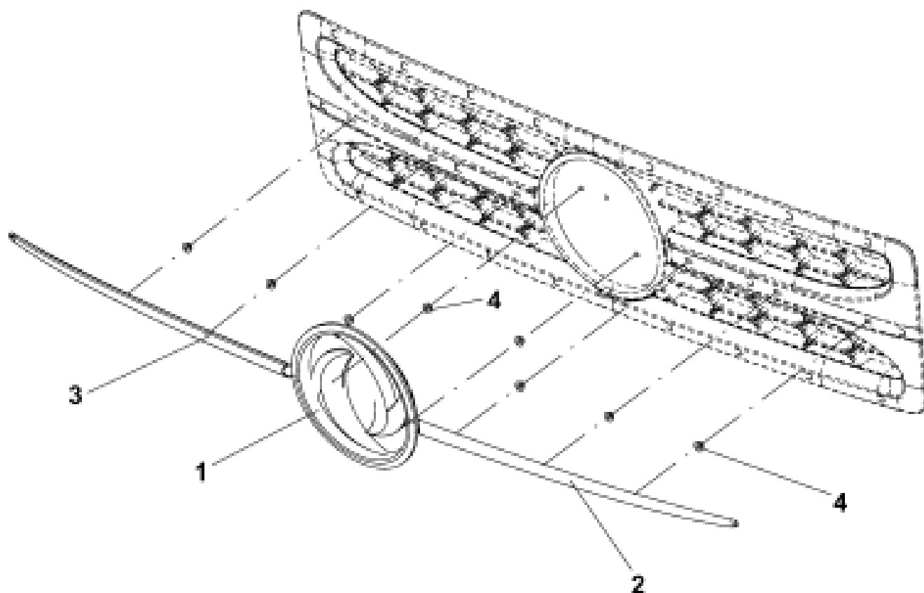
Рис.276. Фирменный знак
