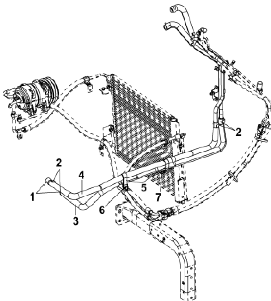
Рис.337. Трубопроводы отопителя
