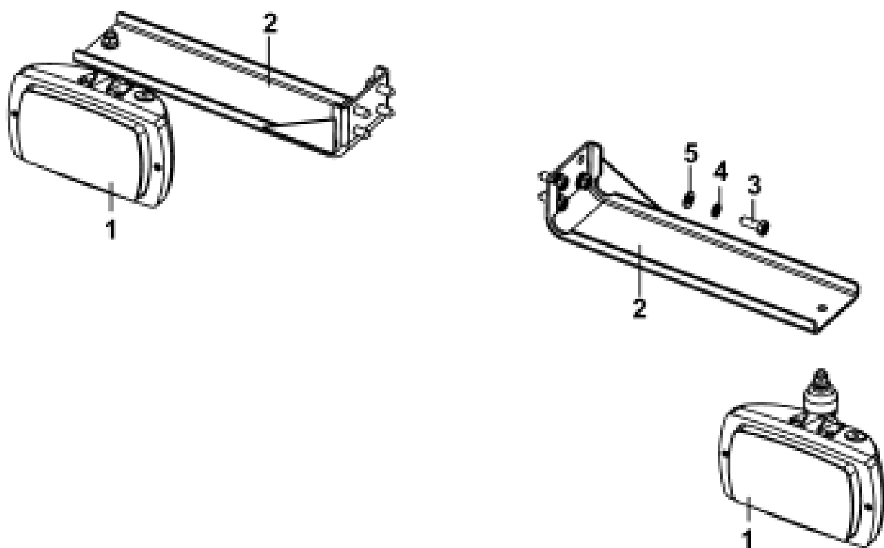
Рис.251. Передние противотуманные фары
