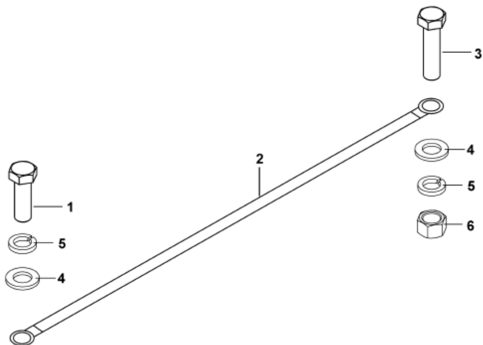
Рис.203. Провод “Масса”
