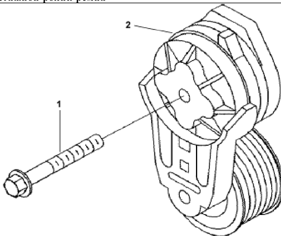
Рис.31. Натяжной ролик ремня
