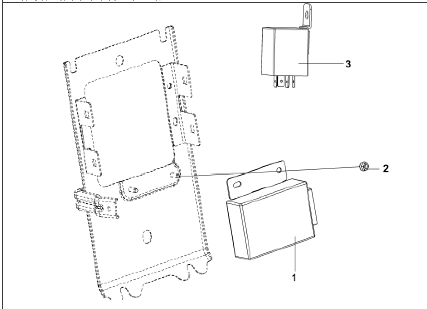
Рис.256. Реле стеклоочистителя
