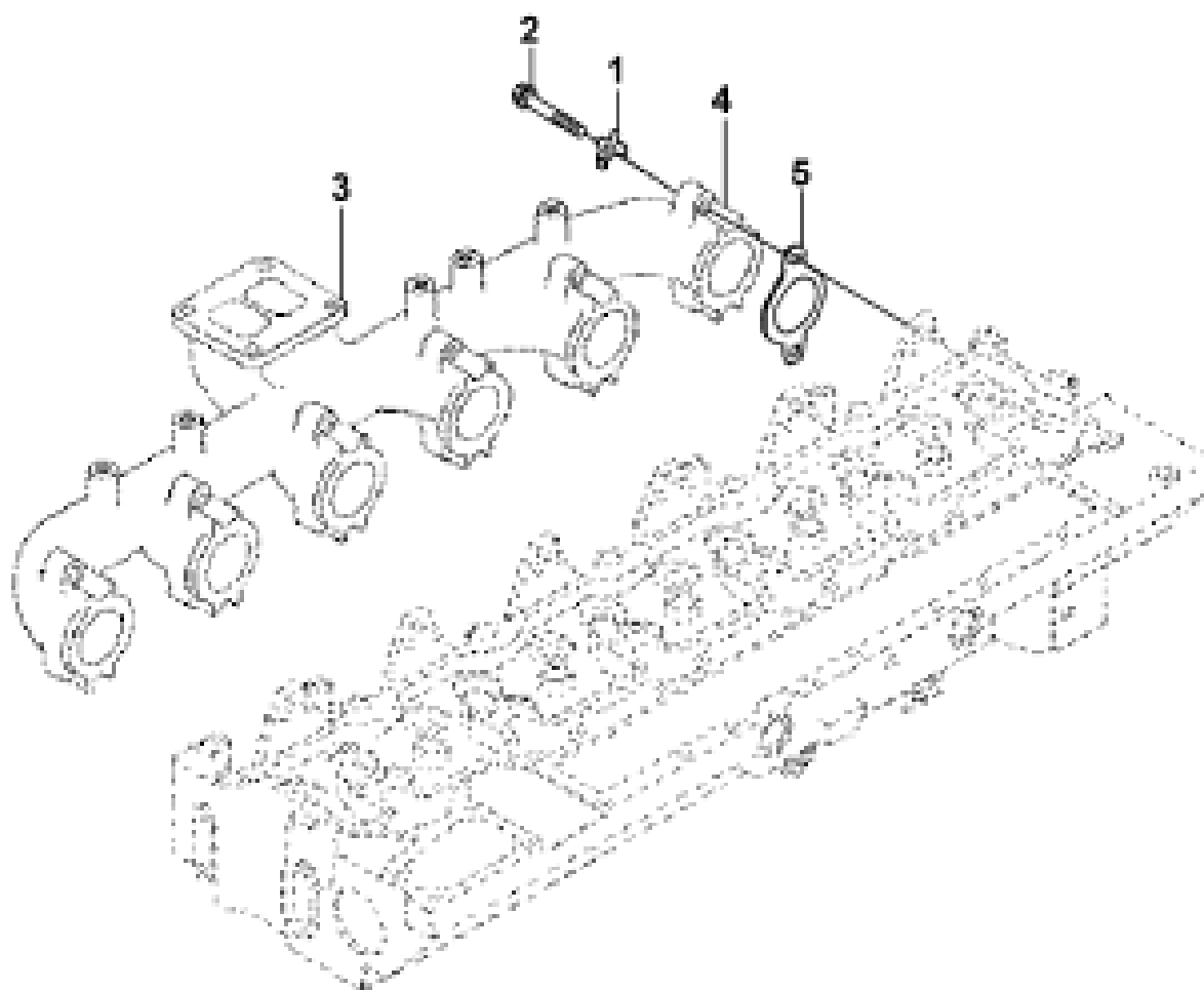
Рис.38. Коллектор выпускной
