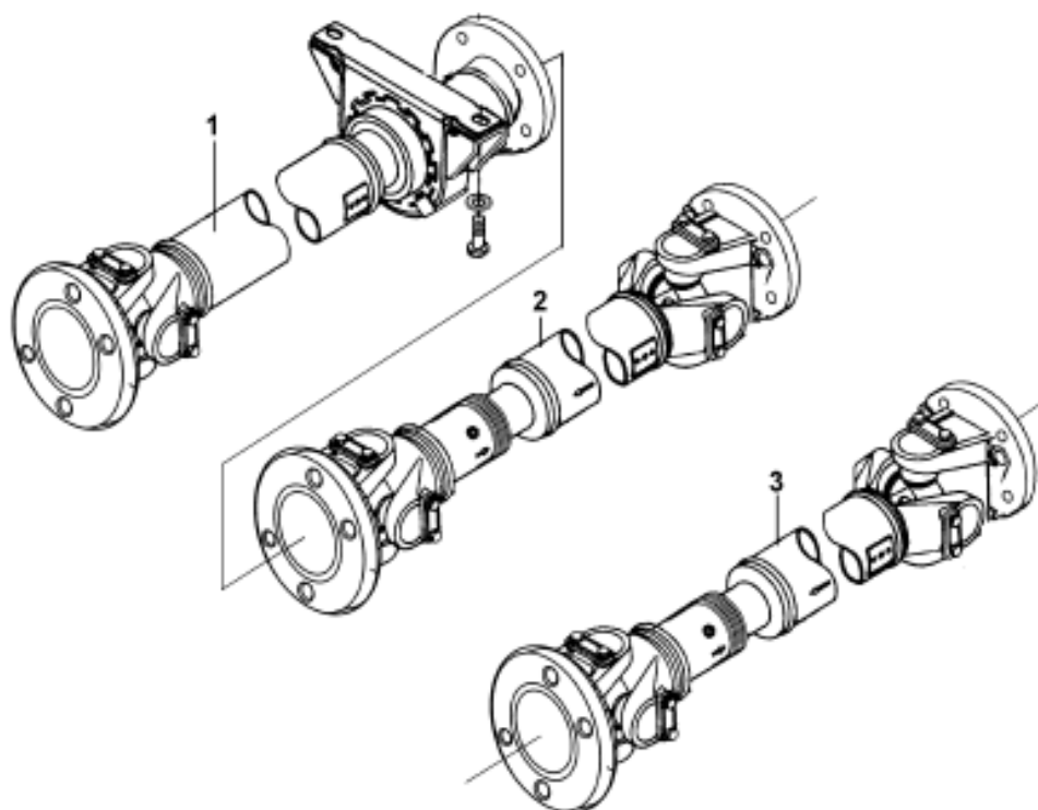
Рис.118. Карданные валы
