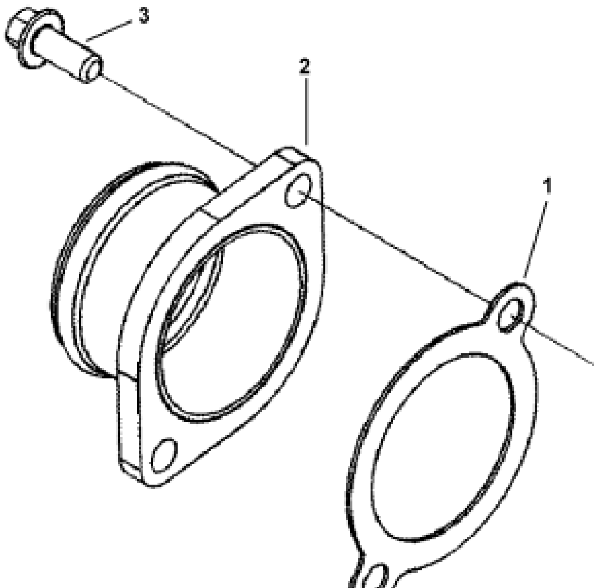
Рис.27. Патрубок
