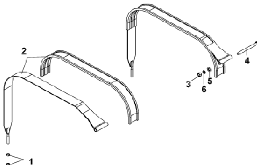
Рис.60. Крепление топливного бака
