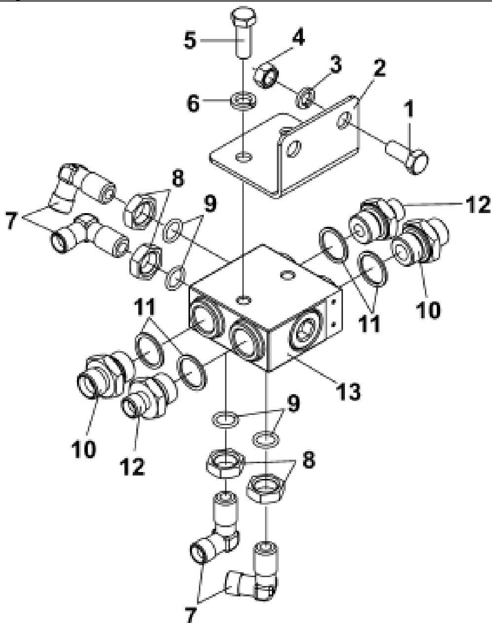
Рис.191. Распределитель
