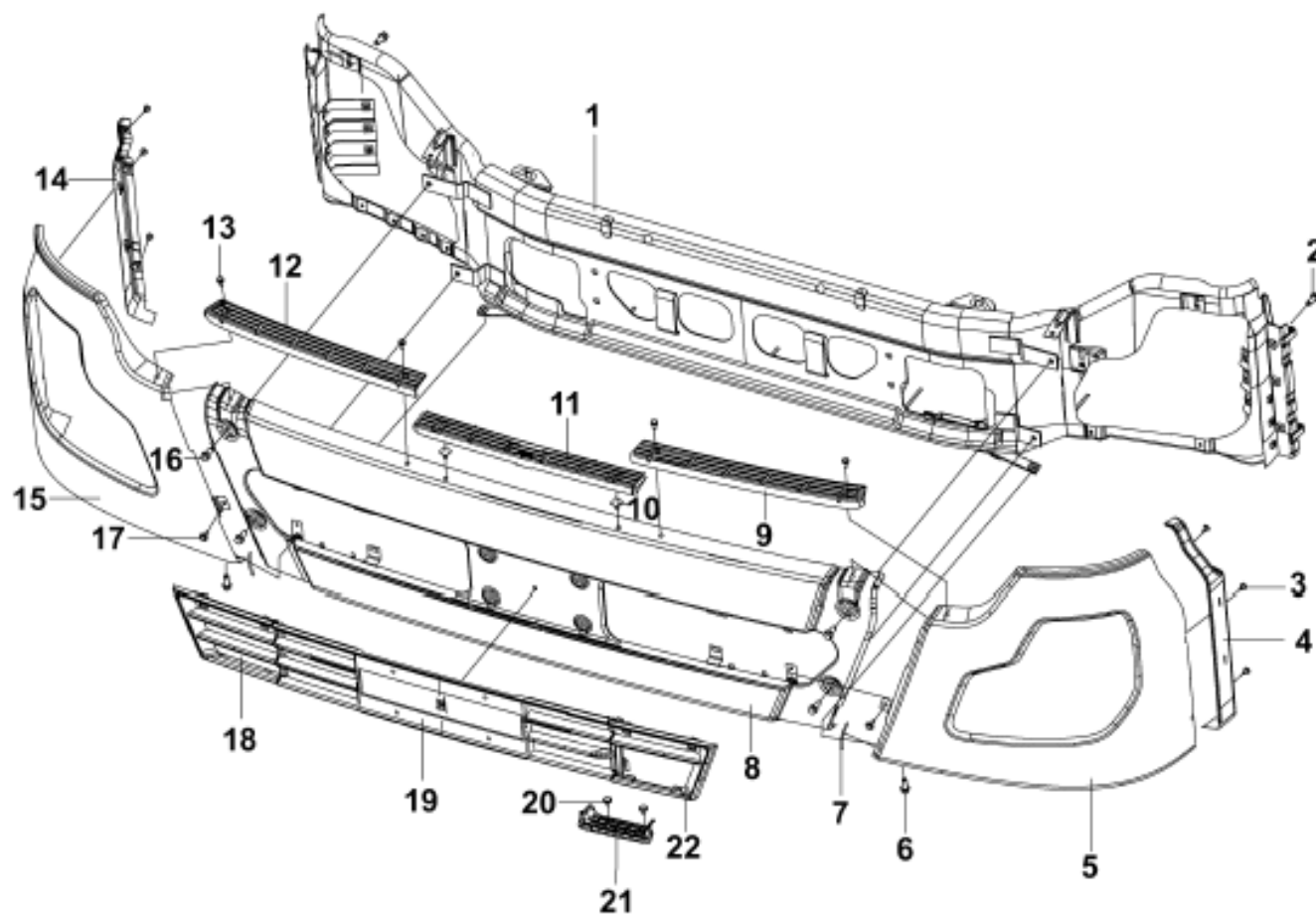
Рис.369. Передний бумер
