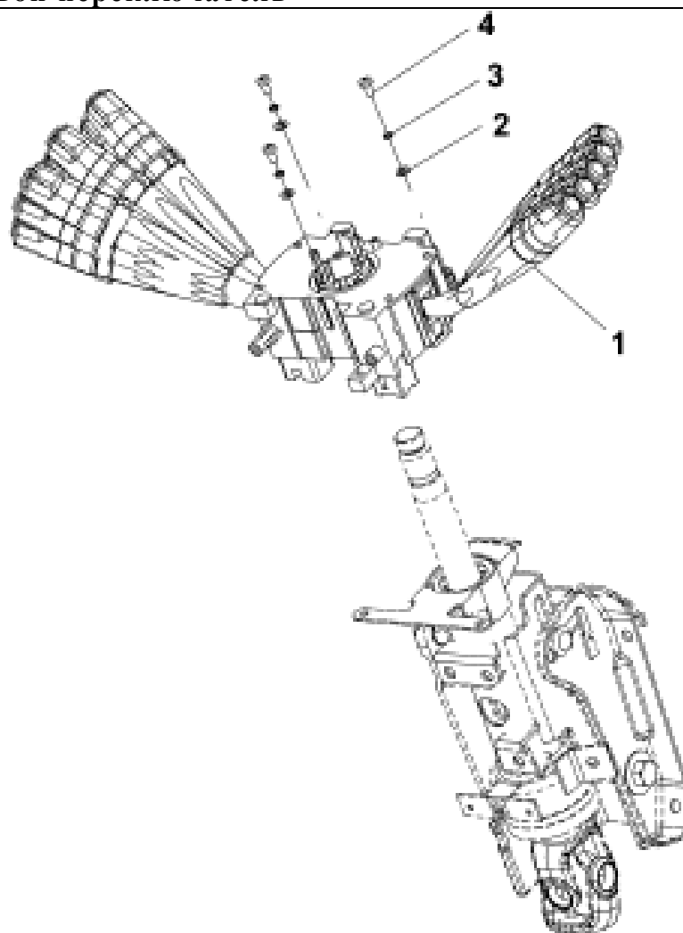
Рис.270. Подрулевой переключатель
