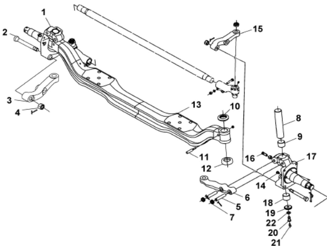
Рис.170. Передний мост
