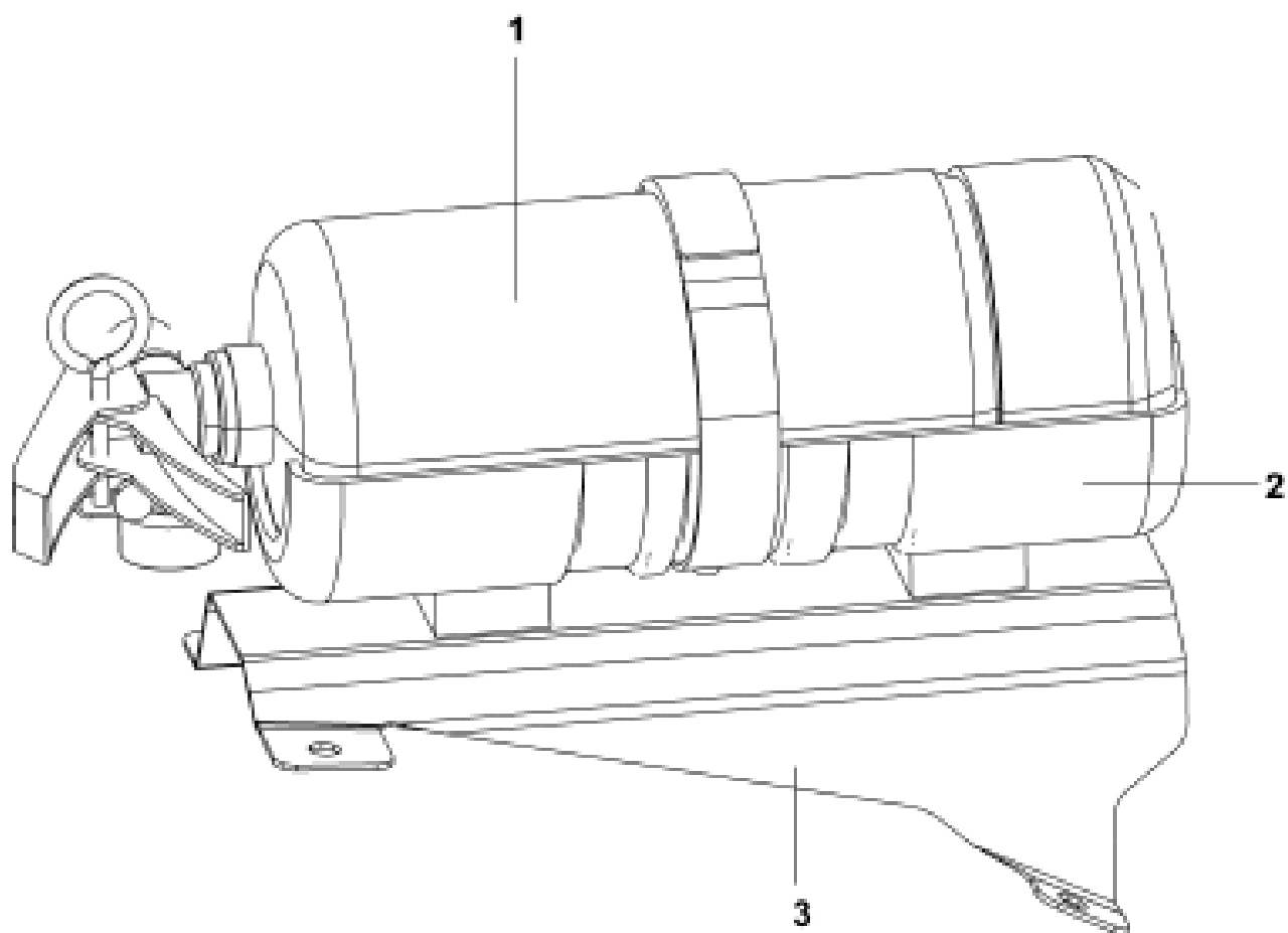
Рис.275. Огнетушитель
