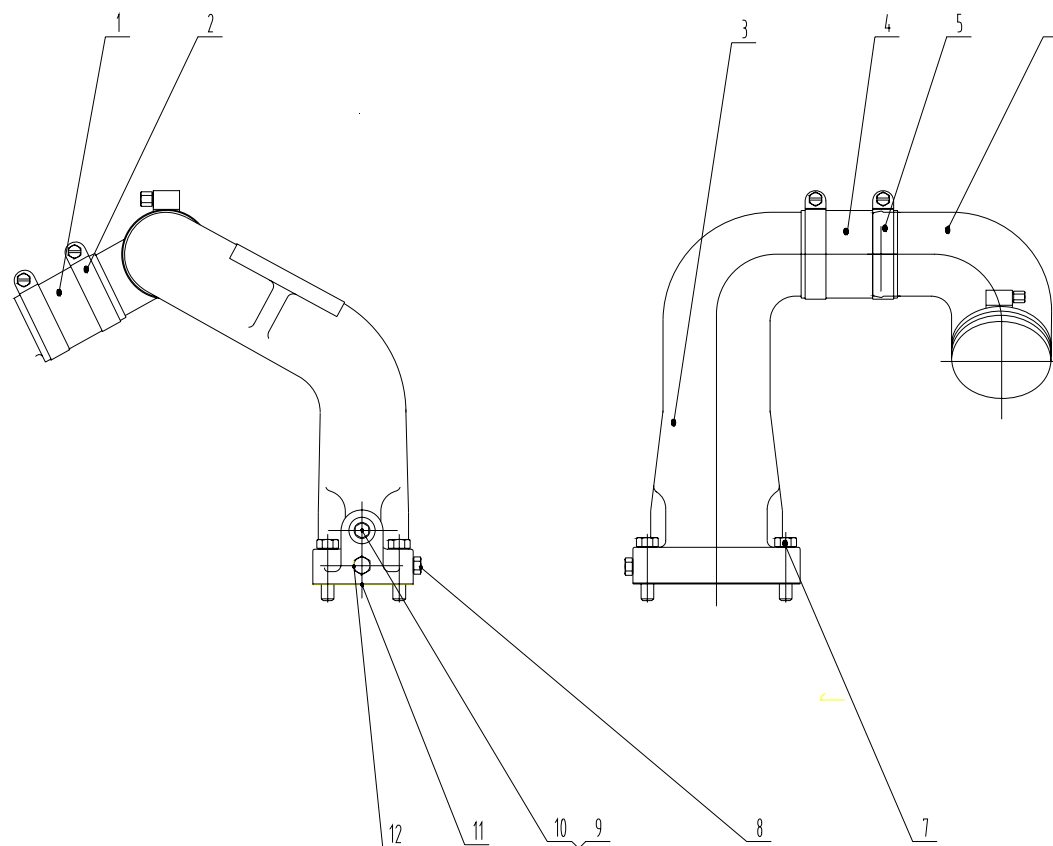
图17 进气管路组件零部件
