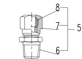
B处局部放大示意图 detail B
